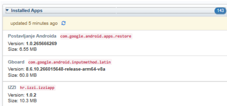
Slika 14. Lista aplikacija koje nisu instalirane kroz MDM sustav
