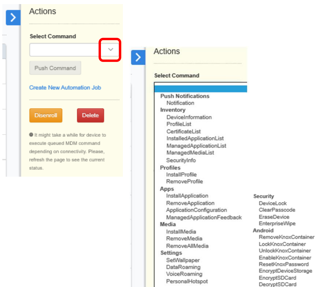
Slika 17. Akcije kojima se šalju razne komande na željeni uređaj
