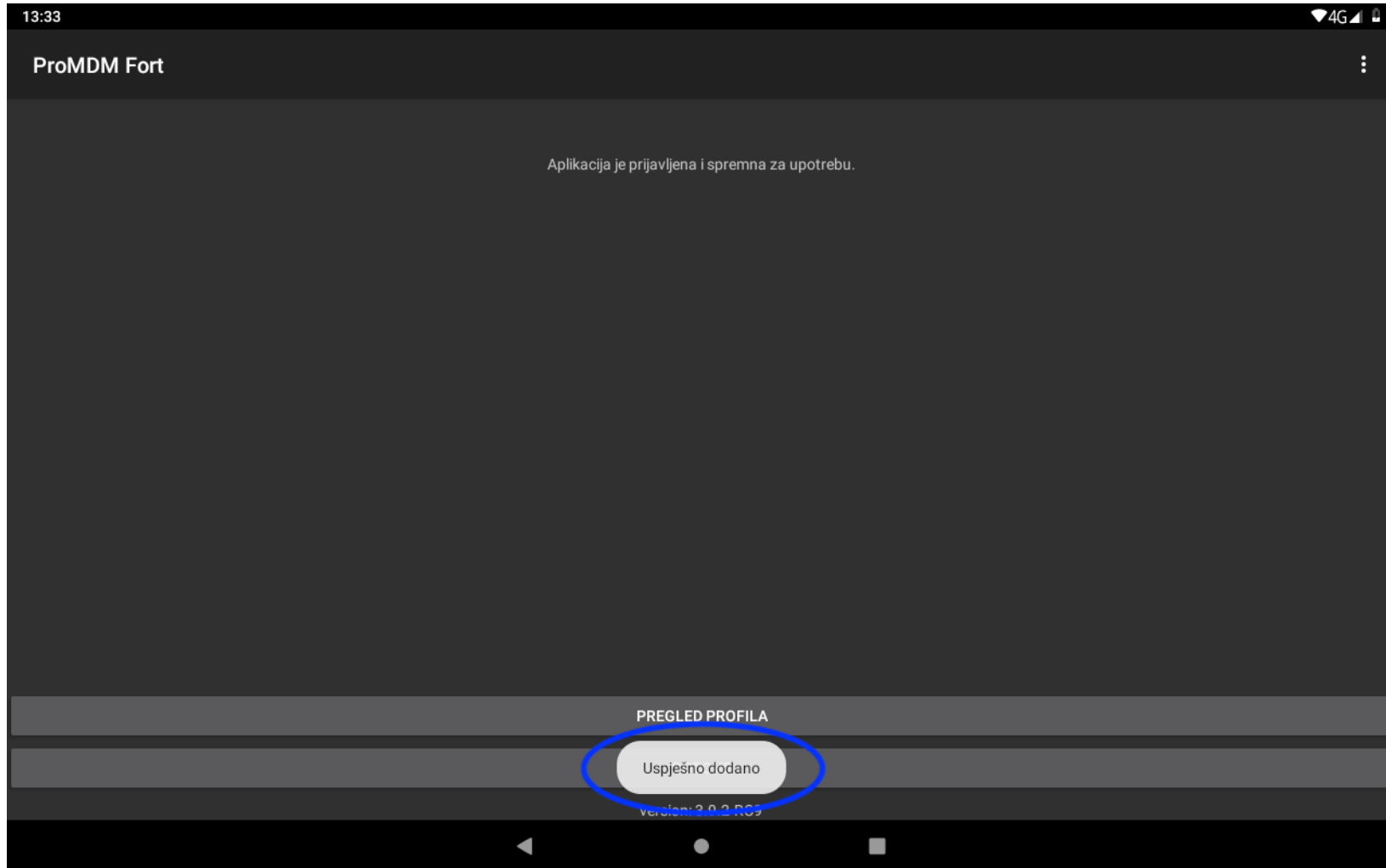
Slika 8. "Uspješno dodano"
