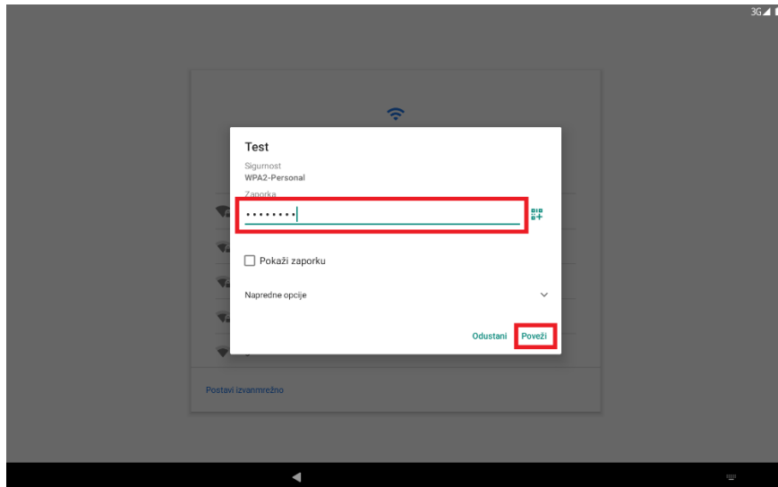
Slika 4. Upisivanje lozinke
