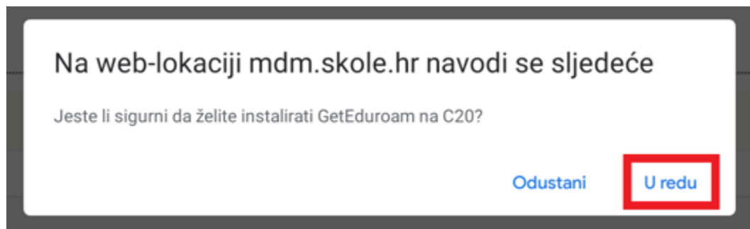
Slika 8. Potvrda instalacije
