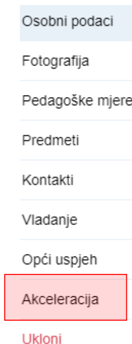
Slika 27 Akceleracija učenika
