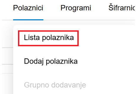
Slika 3. Popis učenika
