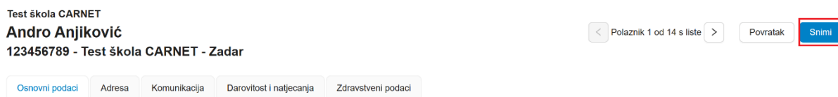
Slika 1. Opcija "Snimi"
